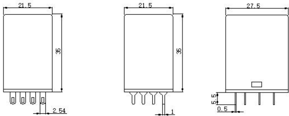
PC Board layout 安装图
